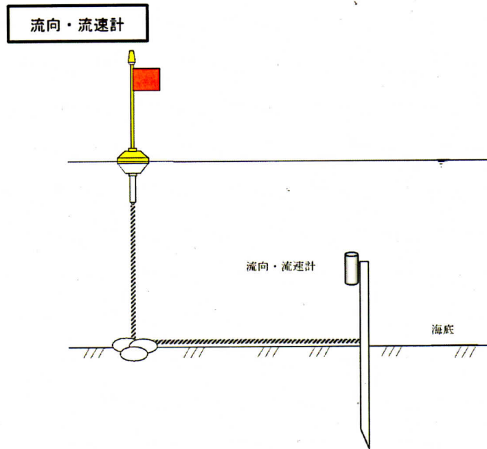
図4 流向・流速計設置概要図
